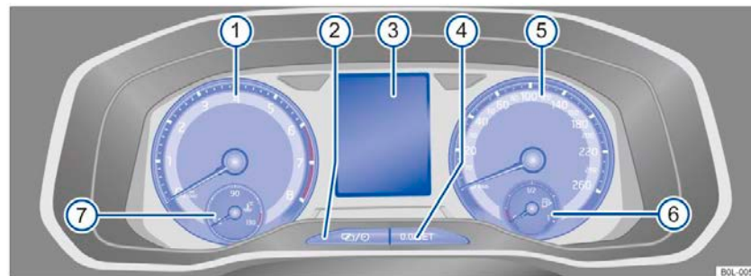
Рисунок 10 Аналоговые приборы на приборной панели (тип II)
