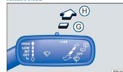
Рисунок 68 Правая сторона рулевой колонки: рабочее положение рычага управления стеклоочистителем заднего стекла
