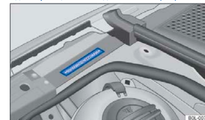
Рисунок 153 В моторном отсеке: Идентификационный код автомобиля (схематическое изображение)
