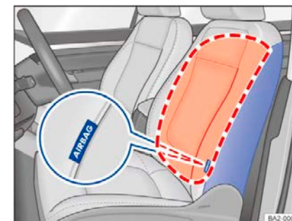
Рисунок 31 Левая сторона переднего сиденья: положение установки и зона действия боковой подушки безопасности
