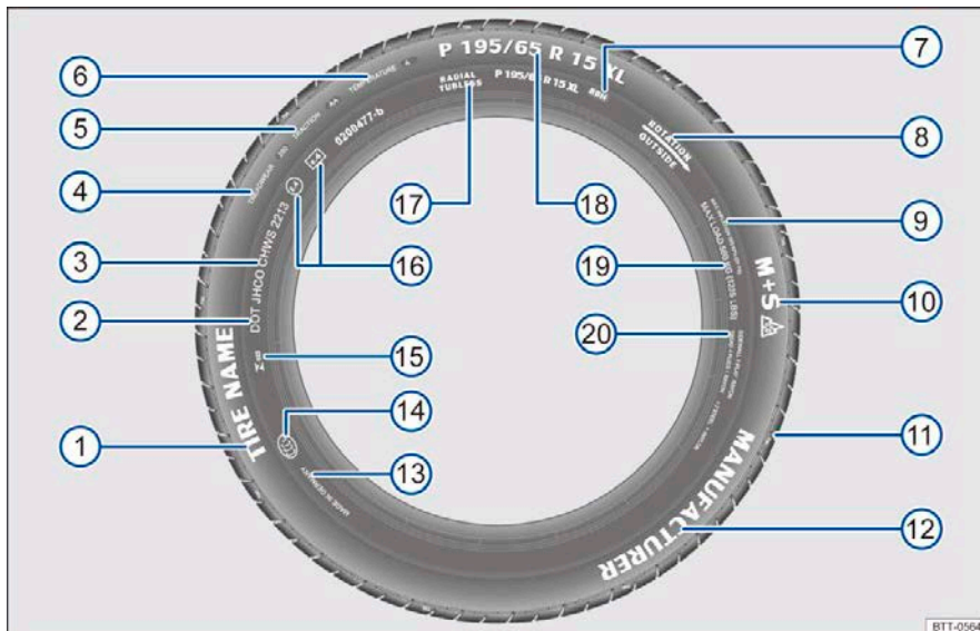
Рисунок 142 Международный общий идентификационный код шин
