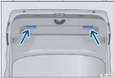
Рисунок 49 Открытая дверь багажного отделения: скрытая ручка для закрывания двери багажника
