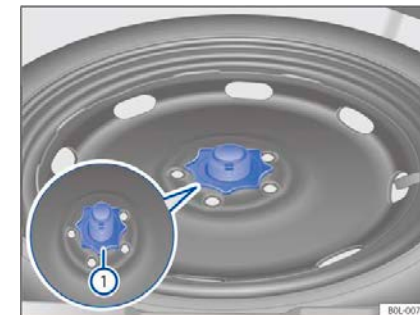
Рисунок 141 В багажнике: маховик для крепления аварийного запасного колеса
