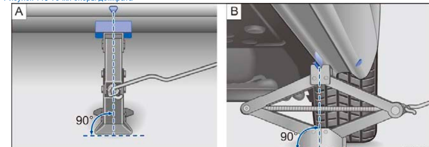
Рисунок 147 Домкрат располагается сзади с левой стороны автомобиля.
