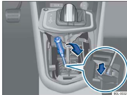
Рис. 87 Ручная разблокировка замка рычага переключения передач
