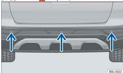
Рисунок 96 На заднем бампере: Ультразвуковой датчик системой предупреждения о превышении дистанции при парковке задним ходом
