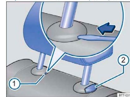
Рисунок 60 Снятие подголовника заднего ряда сидений
