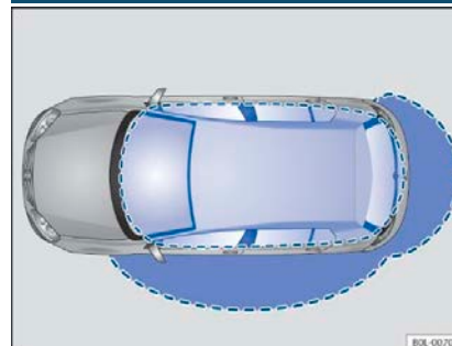
Рисунок 41 Доступ без ключа: зоны срабатывания
