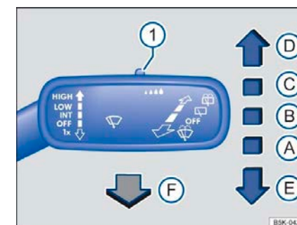
Рисунок 67 Правая сторона рулевой колонки: рабочее положение рычага управления стеклоочистителем лобового стекла
