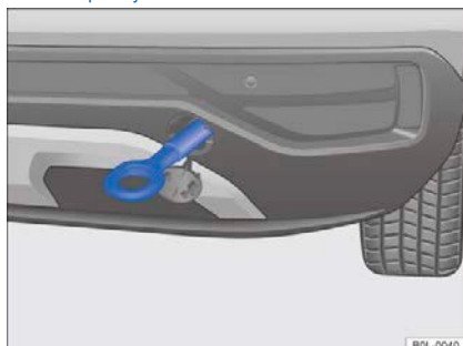
Рисунок 122 Верхняя правая сторона заднего бампера: ввинтить буксирное кольцо Буксирное кольцо должно всегда быть в автомобиле. Обратите внимание на совет по буксировке → стр. 122. Установка заднего буксирного кольца
