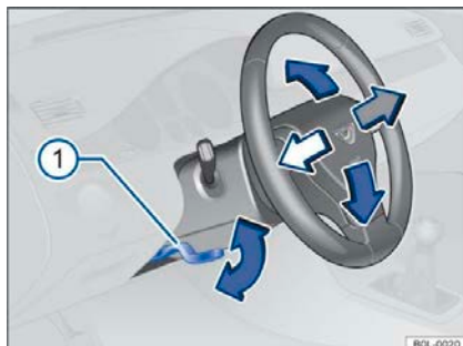
Рисунок 52. На панели обивки рулевой колонки под рулевым колесом: ручка управления механической регулировкой положения рулевого колеса
